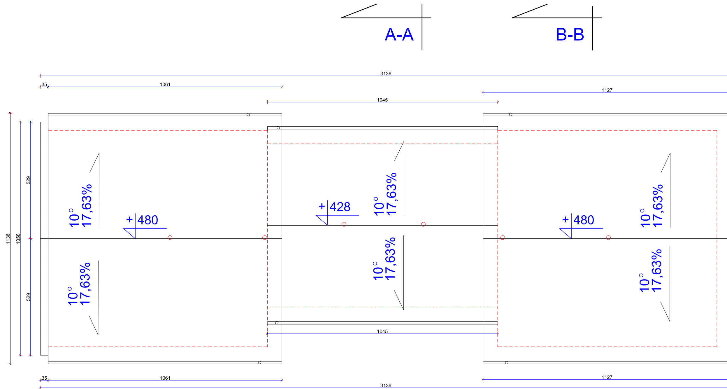
część D magazyn sprzętu rolniczego rzut dachu 1:100
